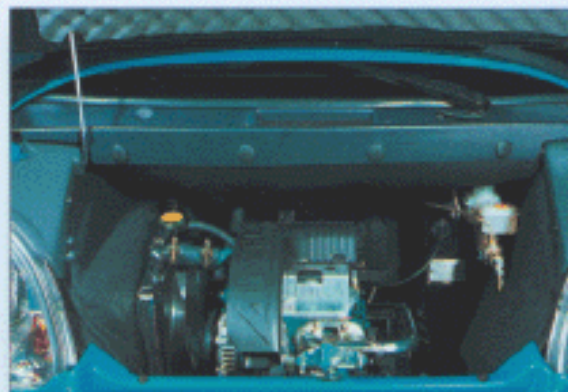
Le moteur KUBOTA spécifique AIXAM et son insonorisation. • Ce moteur a encore progressé en souplesse et en niveau de bruit. • Il respecte largement les normes CEE de pollution. • Sa suspension est étudiée pour limiter les vibrations.
